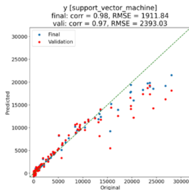
fig. 1: Standard Hyperparameter
